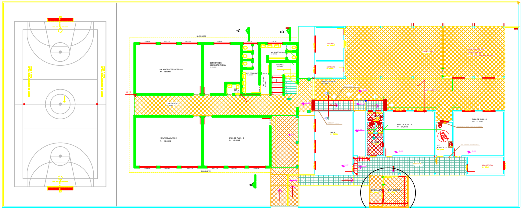
PLANTA BAIXA REFORMA E AMPLIAÇÃO E.R.M. ALMERINDO MANOEL DA LUZ
