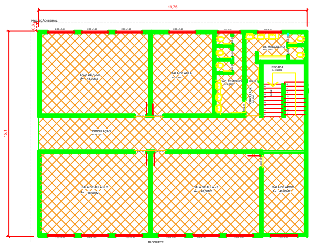
PLANTA BAIXA SEGUNDO PAVIMENTO ÁREA DE AMPLIAÇÃO 298,22 m 2
