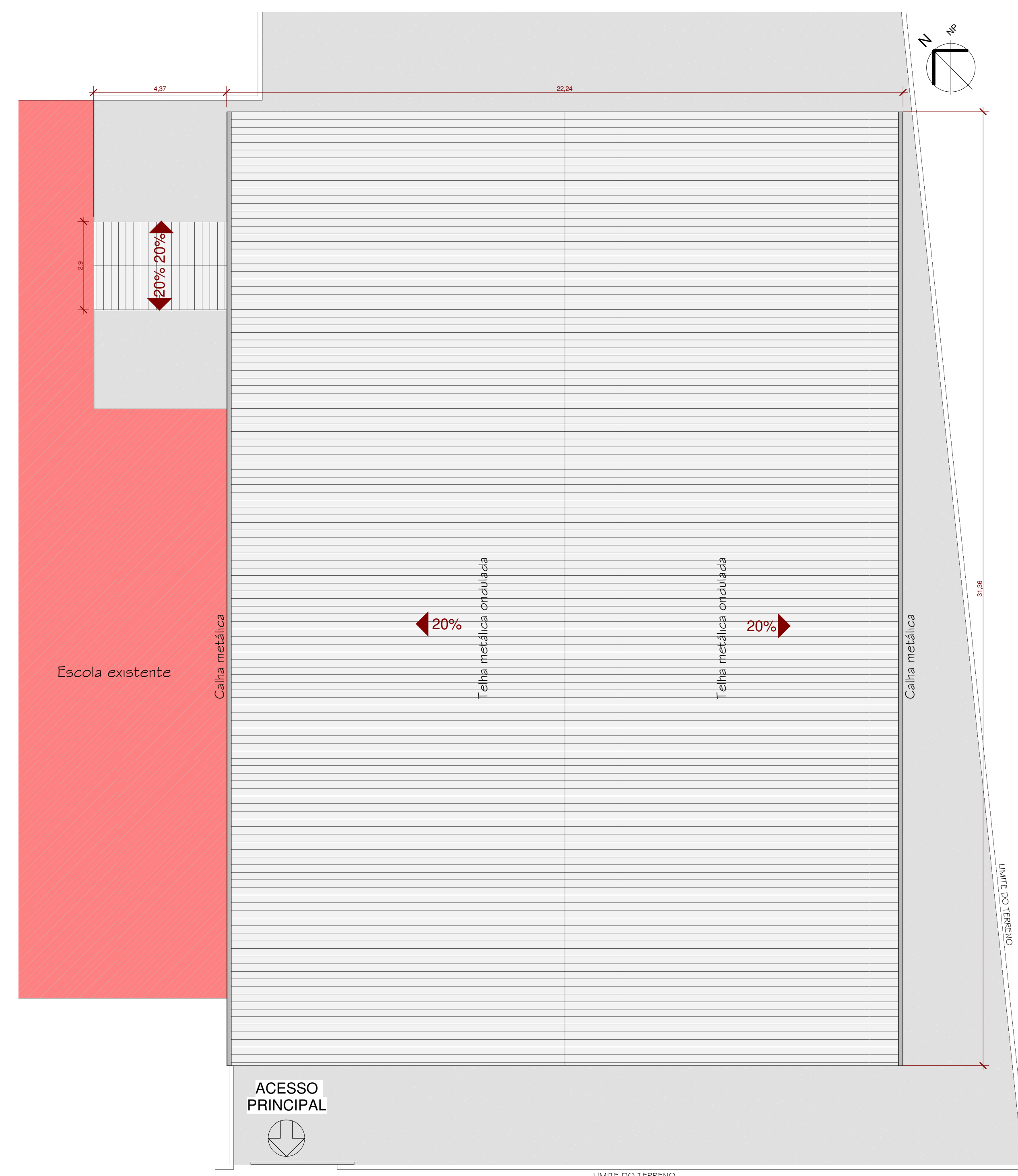
COBERTURA 1:100
