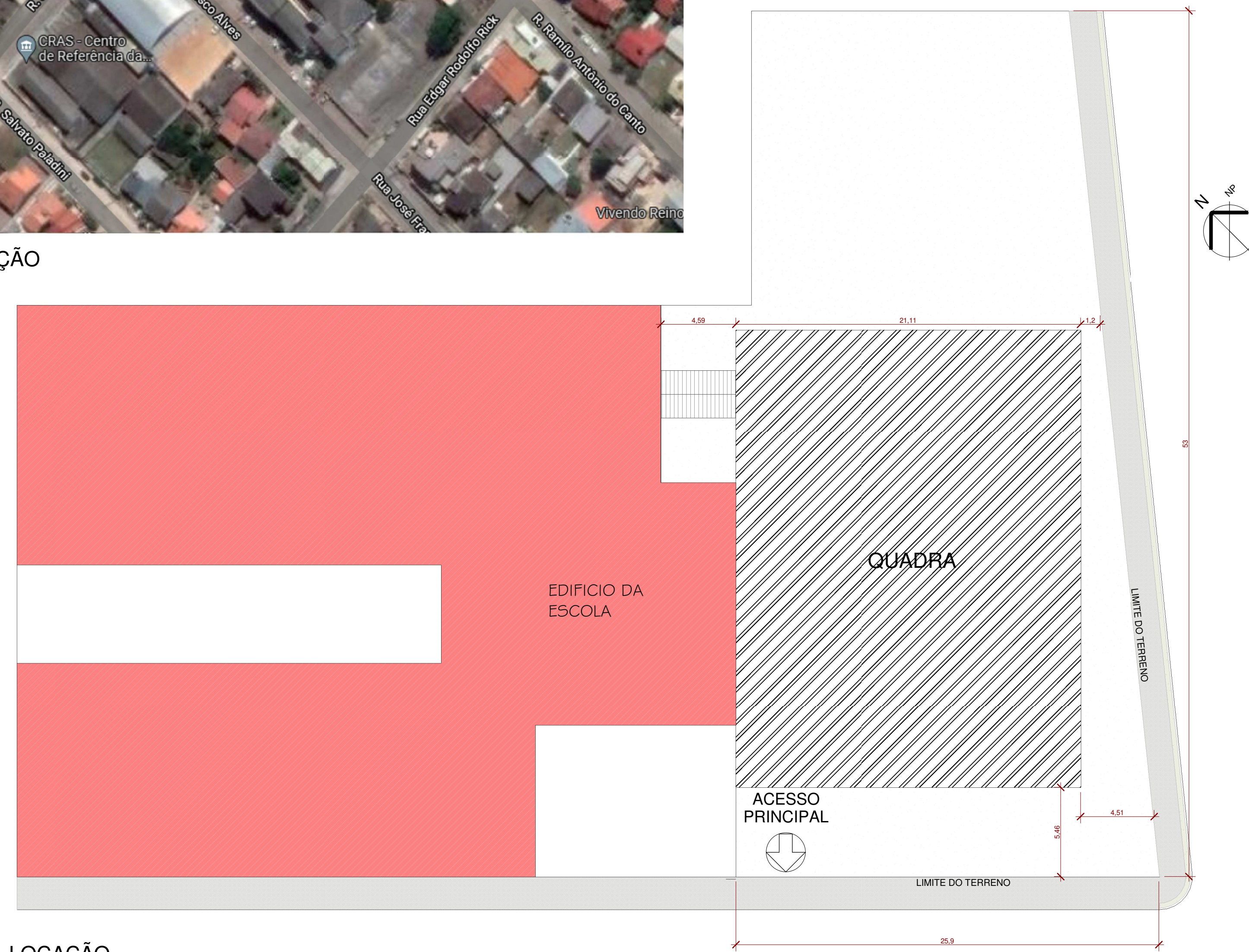
LOCAÇÃO 1:200
