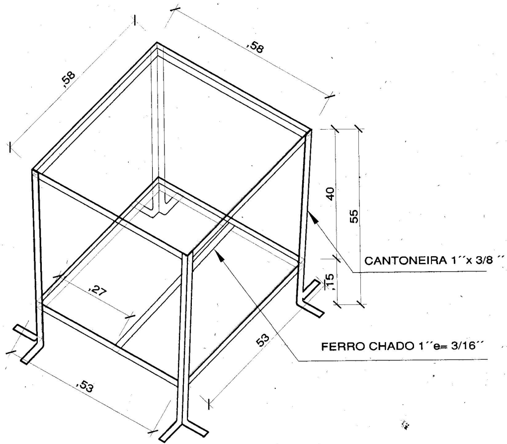
PL. EM PERSPECTIVA
