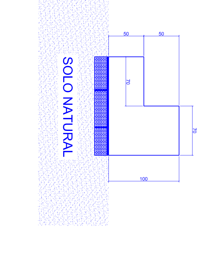
DETALHAMENTO ARQUIBANCADA QUADRA
