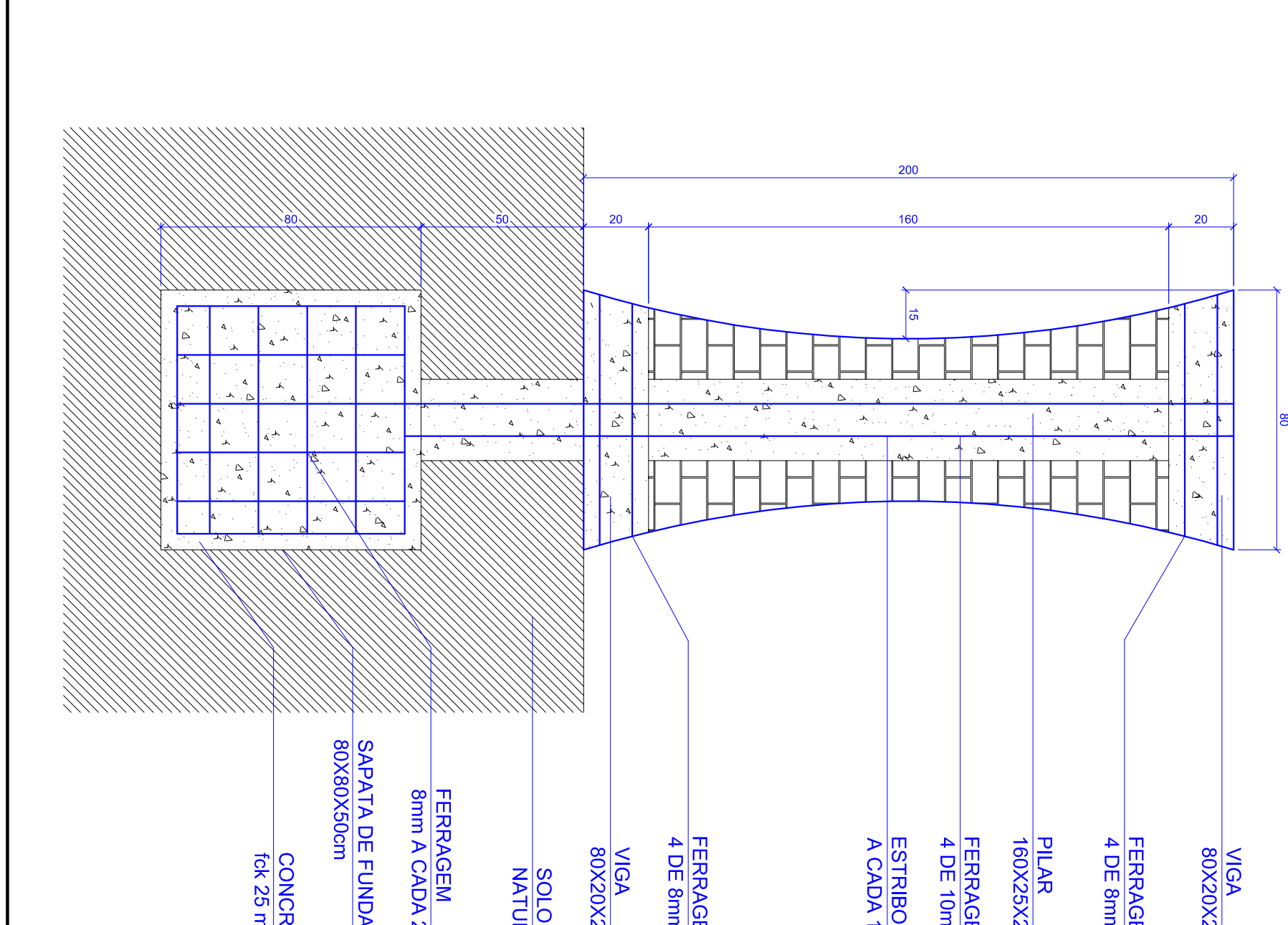
DET. ESTRUTURA TOTEM INFORMATIVO
