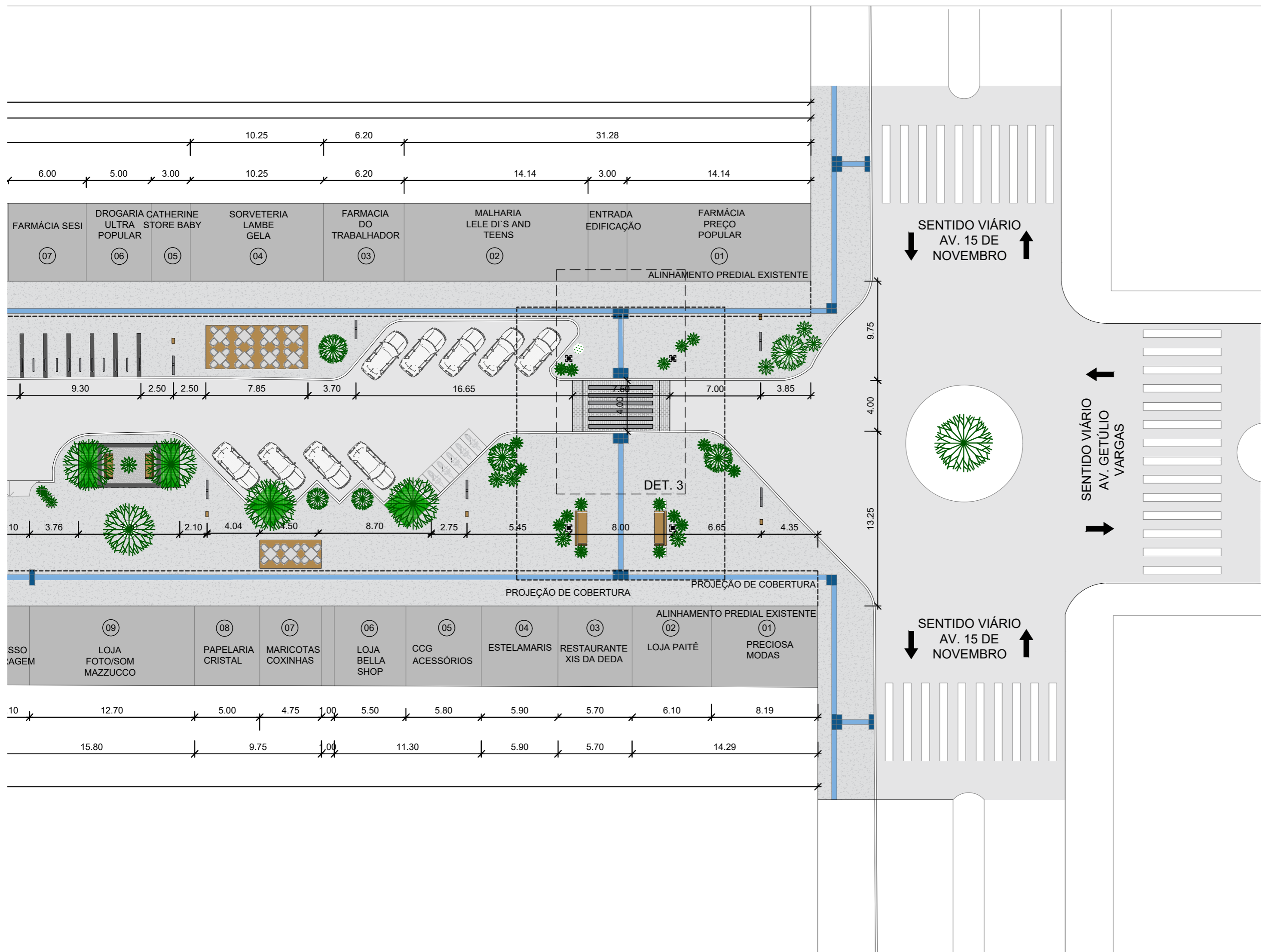
PLANTA BAIXA IMPLANTAÇÃO GERAL - PARTE A ESCALA 1:250
